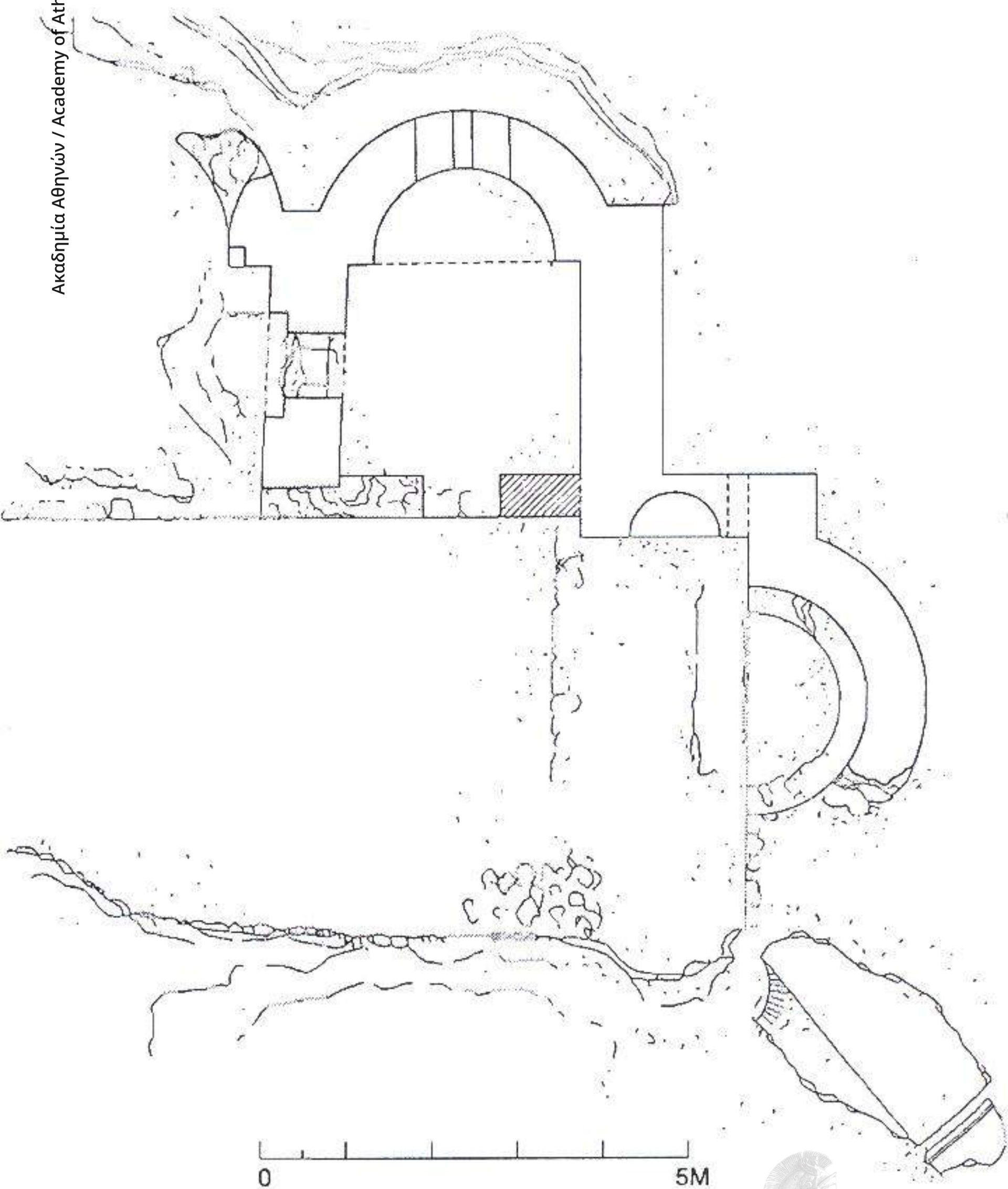
Σχέδ. 1. Κάστρο Ζακύνθου. Ναός Σωτήρος. Κάτοψη. Αποτύπωση (Αύγουστος 2005).
