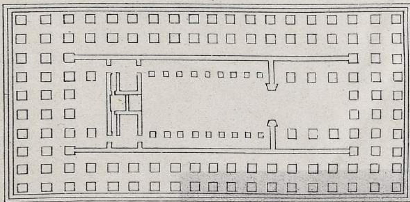
Ναὸς ὀρειόλεως, δωδύλεως, Ὀλύμπιος
