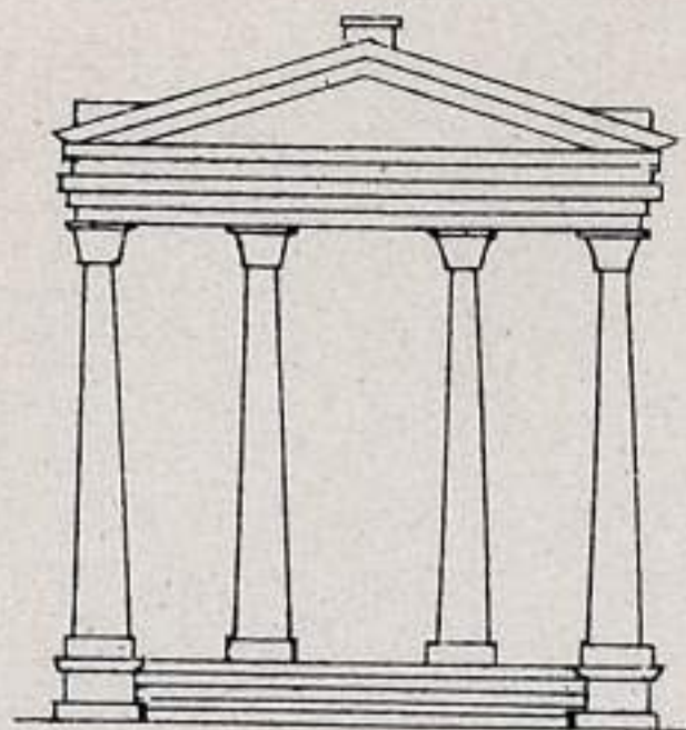
Ναὸς ἀμφωροδόλυφος, τετραδόλυφος Πρόσοψη
