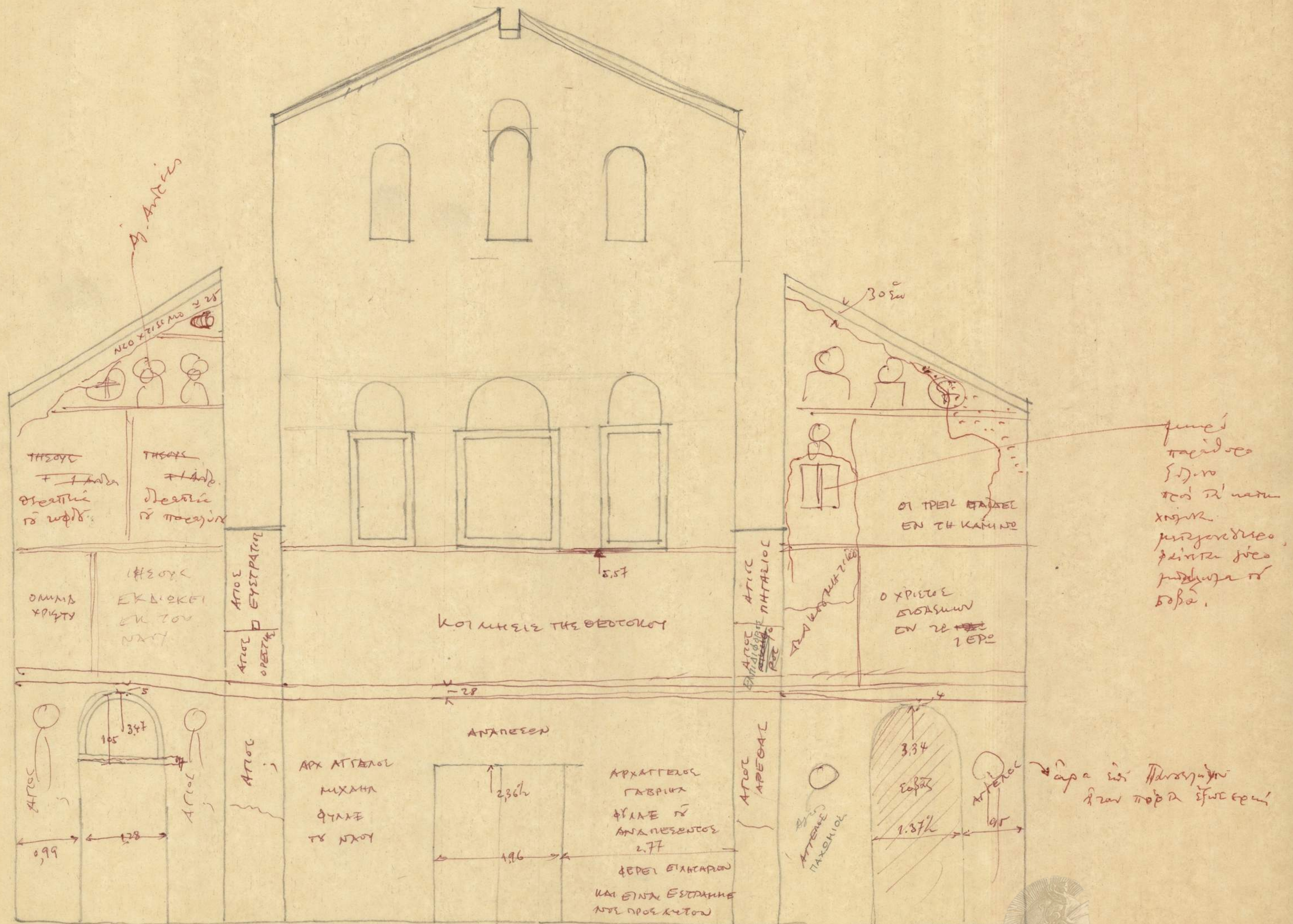
ΕΓΚΑΡΕΙΑ ΤΟΜΗ ΕΙΣ ΤΑ ΔΙΑΜΕΡΙΣΜΑΤΑ Γ.Β.Α., ΒΛΕΠΟΥΣΑ ΠΡΟΣ ΔΥΣΜΑΣ Δ3-Δ3, Π.ΜΥΛΩΝΑΣ, 1971
