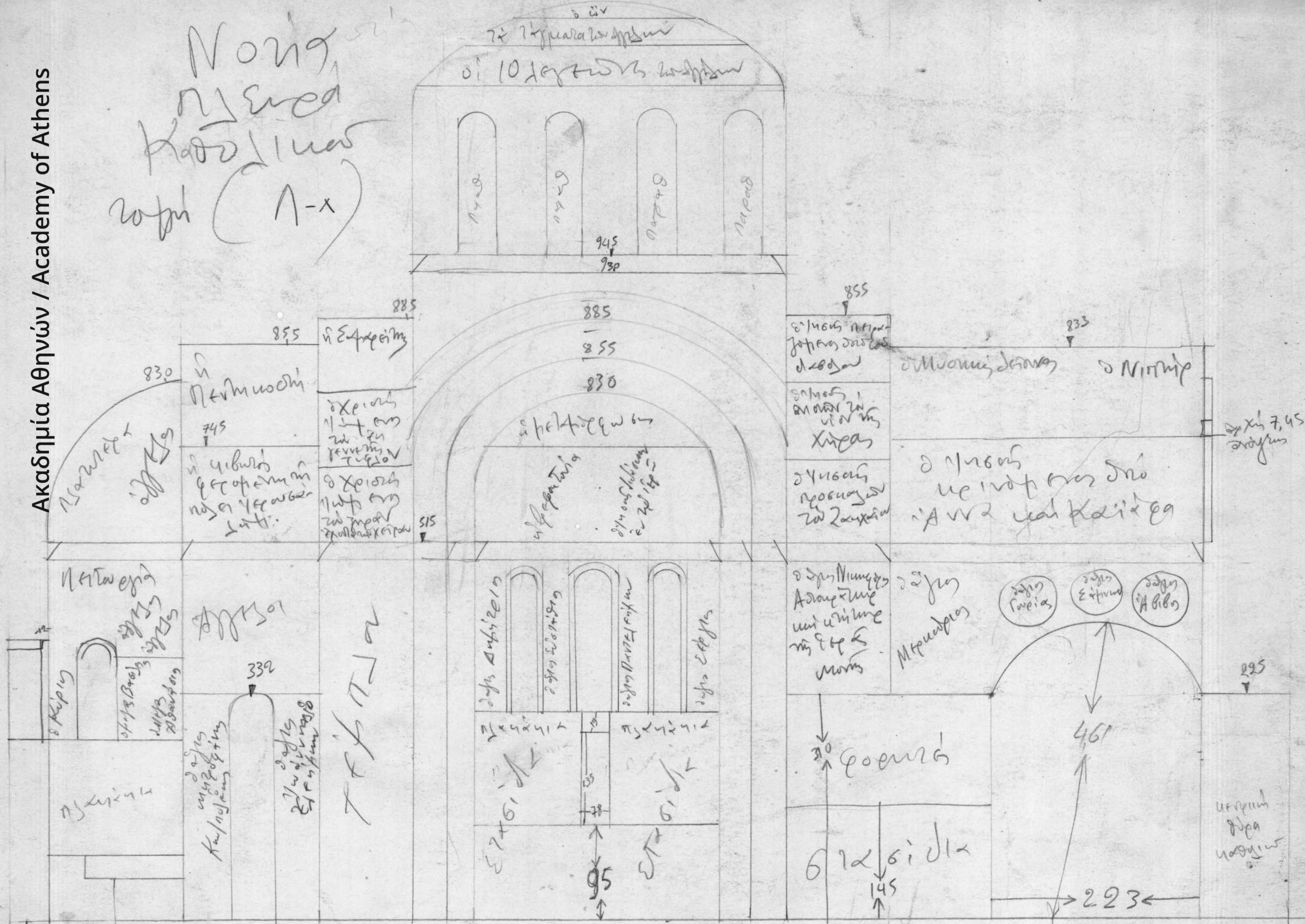
ΝΟΤΙΟΣ ΤΟΙΧΟΣ ΤΗΣ ΚΑΤΑ ΜΗΚΟΣ ΤΟΜΗΣ Α-Α ΜΙΧ ΟΙΚΟΝΟΜΙΑ Η΄, ΝΟΕΜΒΡΙΟΣ 1971
